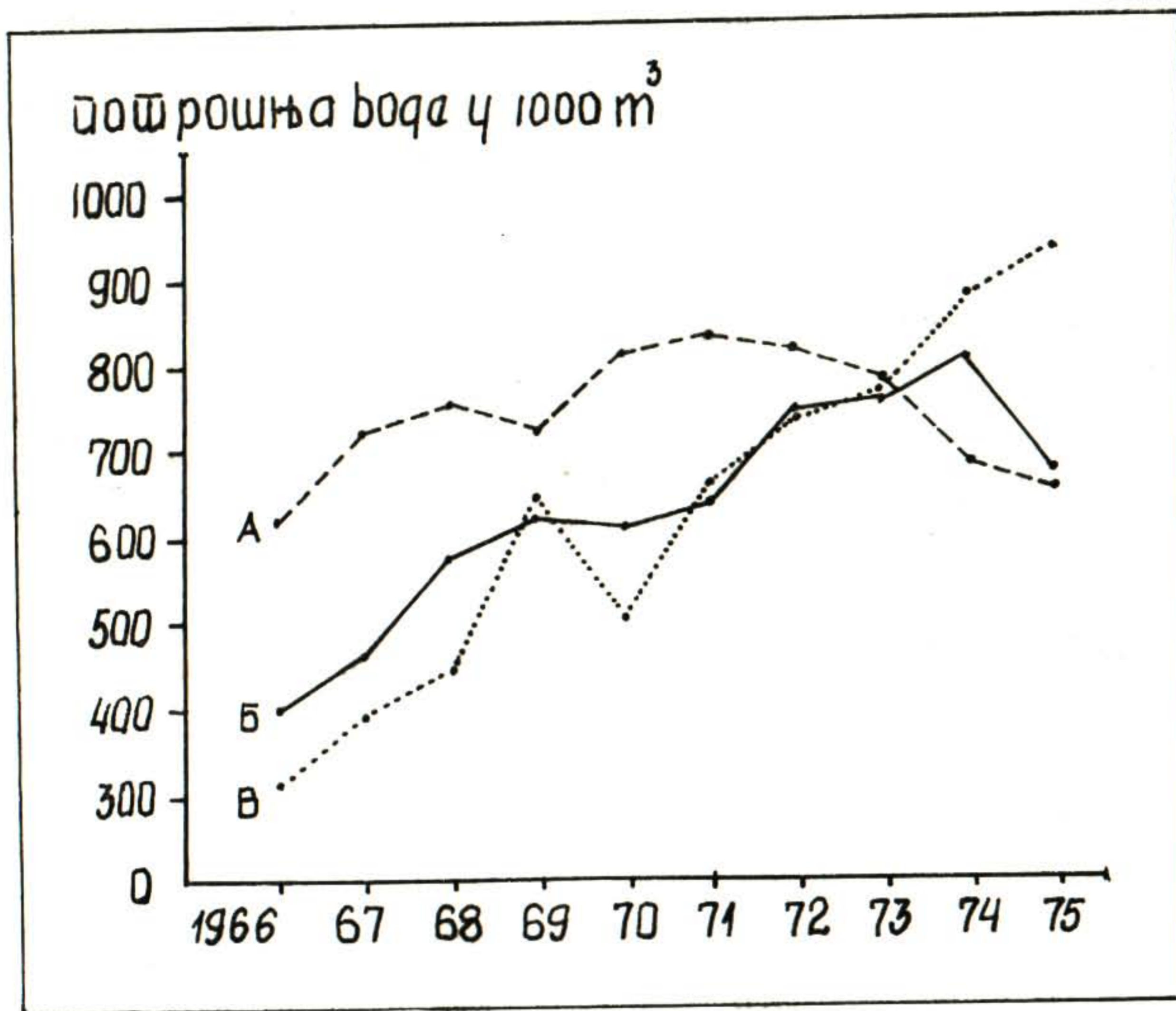
Сл. 2. Кретање потрошње воде: Памучног комбината (А), предузећа и установе (Б), градског становништва (В).
